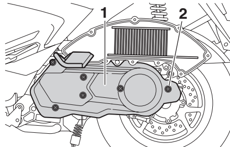
1. V型皮帶箱空氣濾清器蓋 2. 螺絲(x6)
