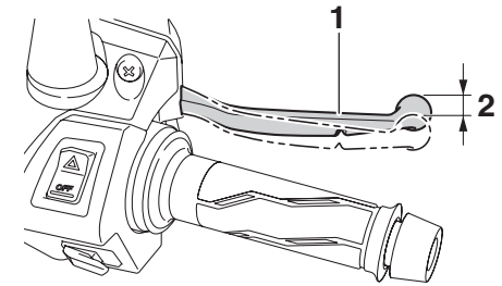
1. 前煞車把手 2. 自由間隙
