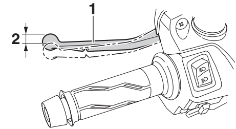
1. 後煞車把手 2. 自由間隙
