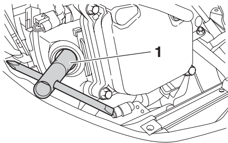
1. 火星塞扳手
