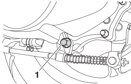
1. 排油螺栓
