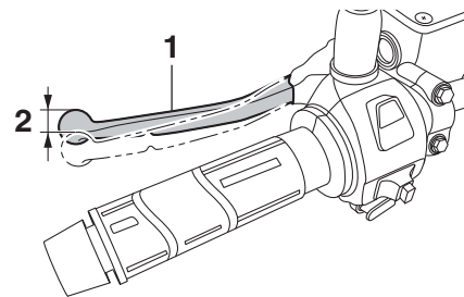
1. 後煞車把手 2. 後煞車把手自由間隙
