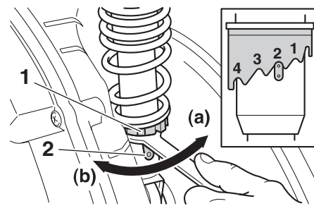
1. 彈簧預載調整環 2. 位置指示器
