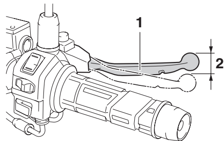
1. 前煞車把手 2. 前煞車把手自由間隙
