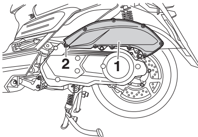
1. 空氣濾清器箱蓋 2. 螺絲(x9)
