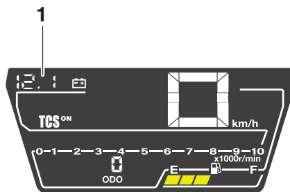
1. 即時電壓
