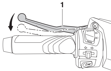
1. 後煞車把手
