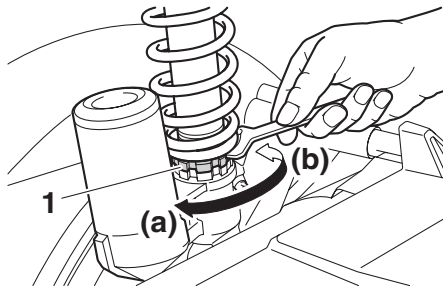
1. 調整環
