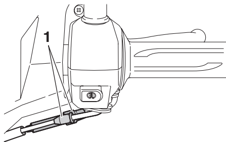
1. 防塵橡皮套
