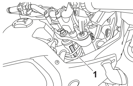
1. 車體號碼
