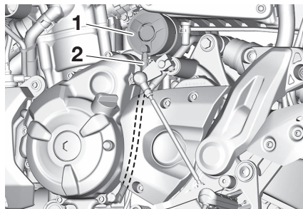
1. 蒸發排放活性碳罐 2. 碳罐通氣軟管
