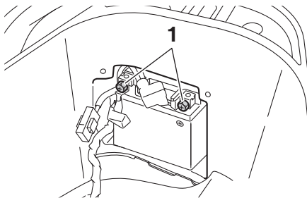
1. 固定螺栓(x2)
